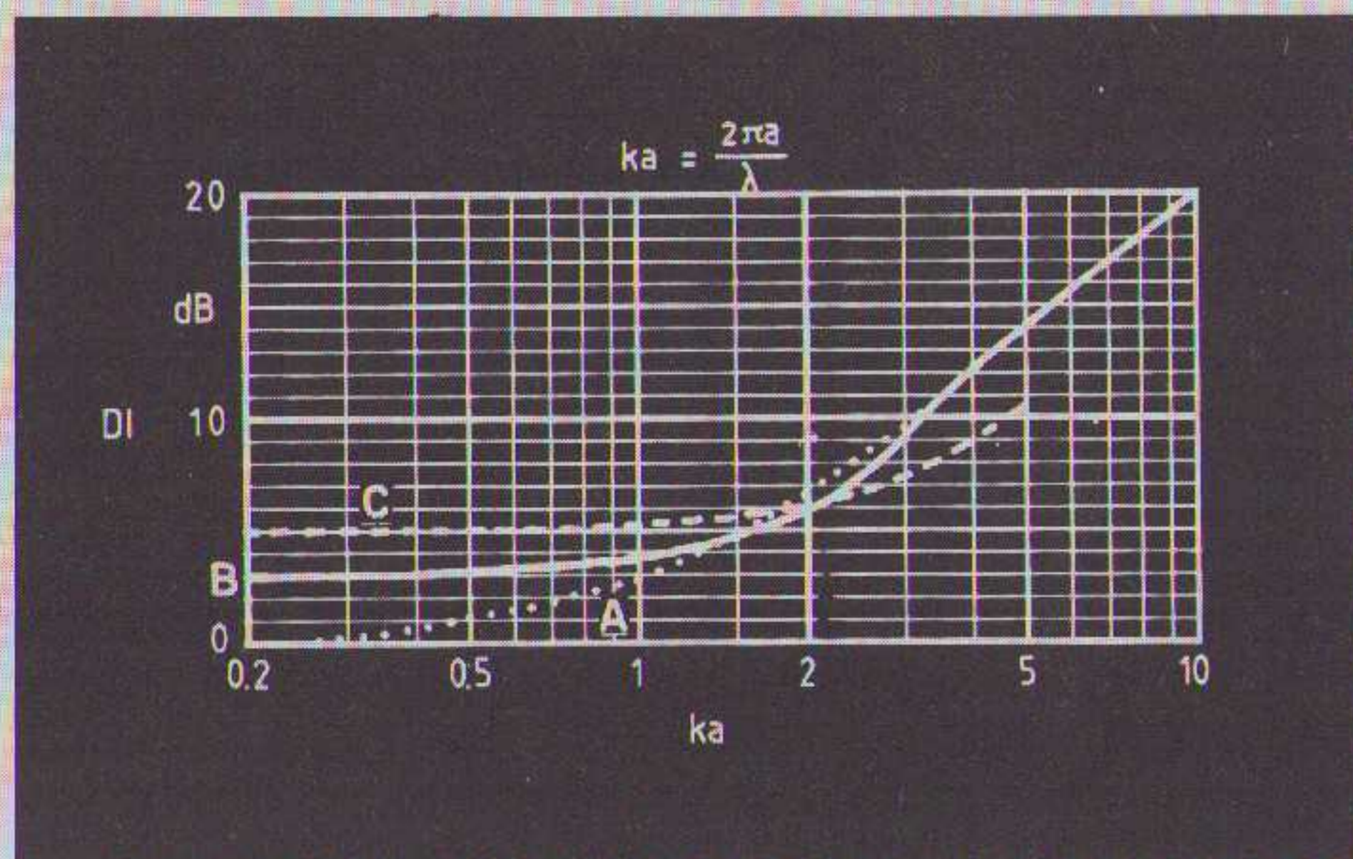
Fig. 46. Directivity index kan een stijve cirkelvormige zuiger als functie van ka = \text{omtrek} / \text{golflengte} . A: aan het eind van een zeer lange buis B: in een oneindig groot klankbord C: vrij in de ruimte.
